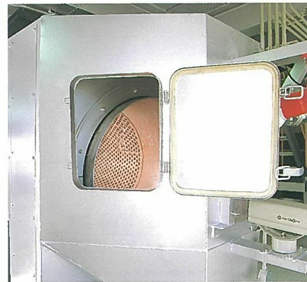
可燃物不燃物選別機(トロンメル)
